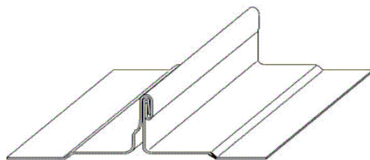
Doppelstehfalz mit Clip Relief
